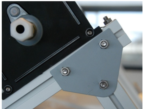
3. Monteer (nr. 1) profielstaander voorzijde aan (nr. 2) profielstaander achterzijde en gebruik hiervoor (nr. 6) de 45° driehoek verbindingplaat. (Zie foto rechtsboven)
